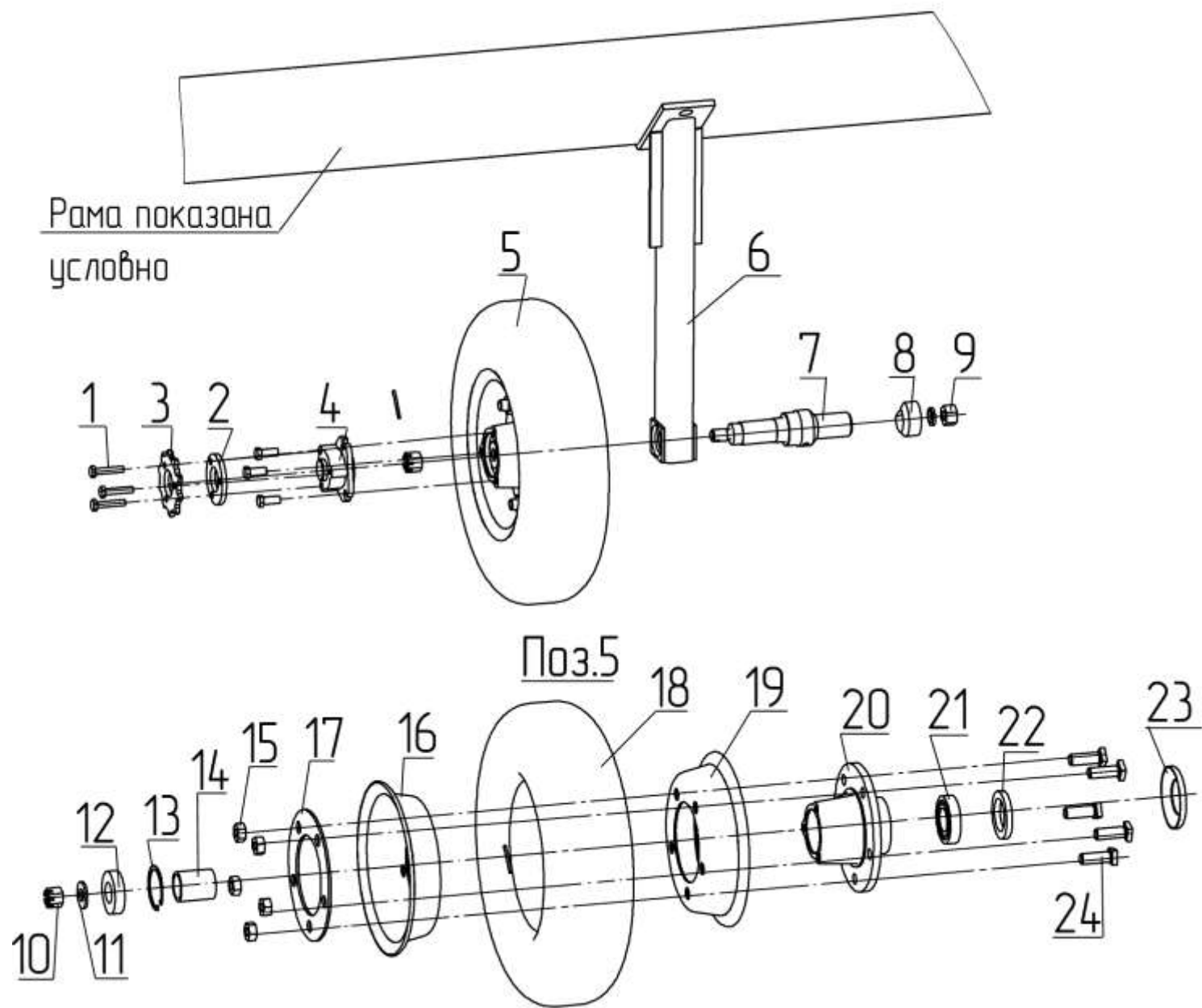
Рис.5 – Колесо КРНВ 46.070
