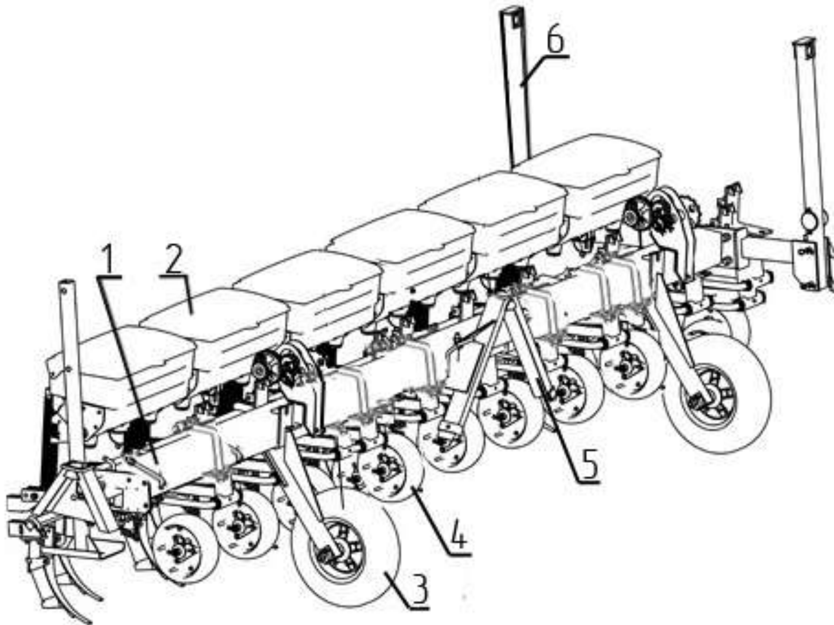
Рис.1 – Культиватор навесной для высокостебельчатых культур КРНВ-5,6-02
