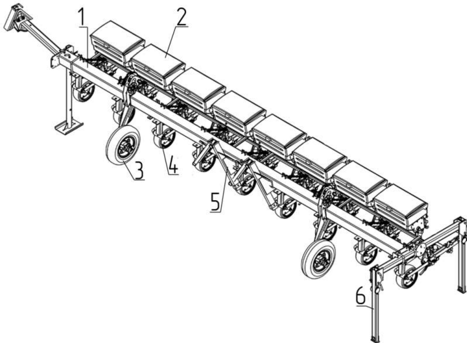
Рис.2 – Культиватор навесной для высокостебельчатых культур КРНВ-5,6-04
