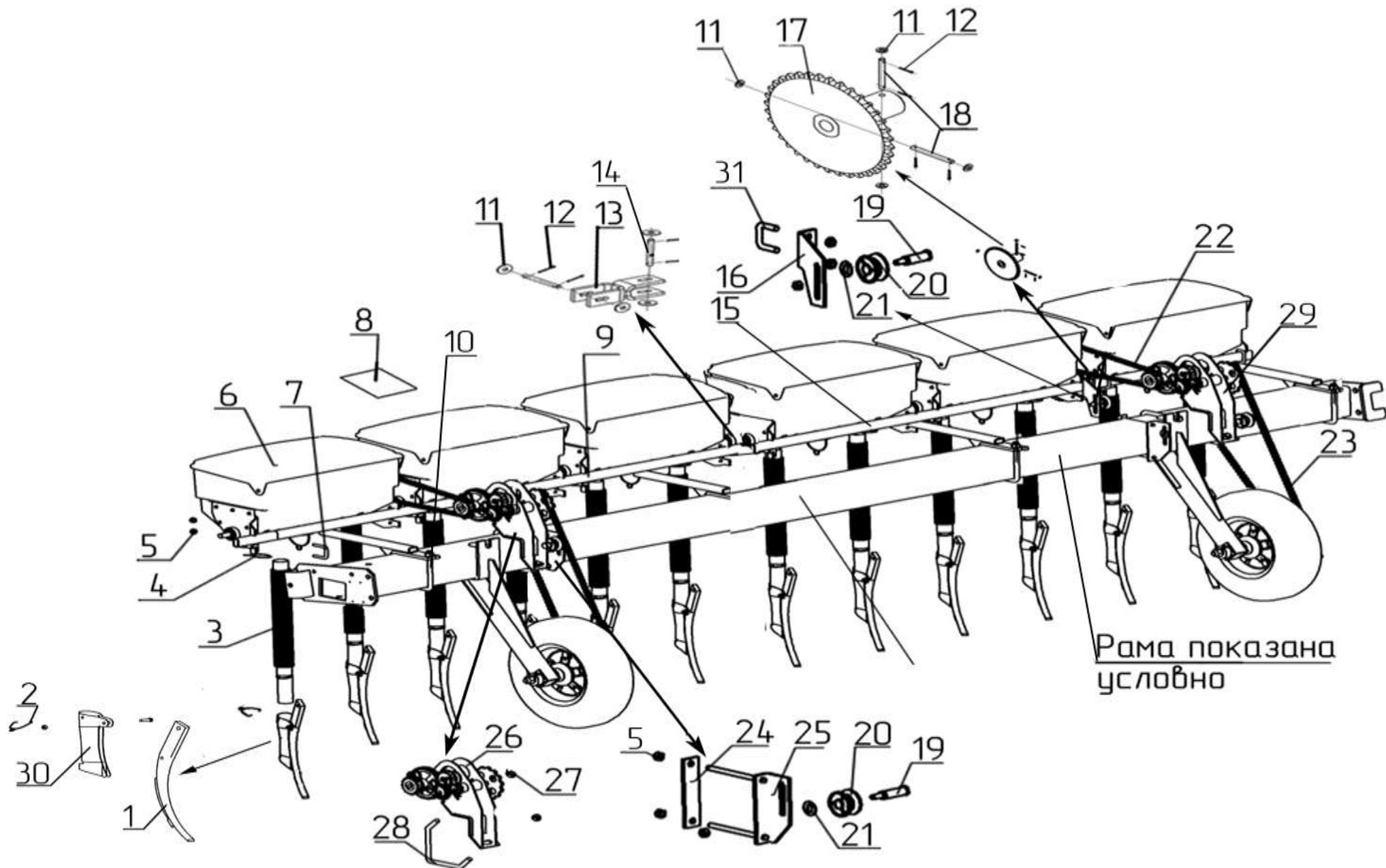
Рис.7 – Подкормочное приспособление КРН 46.380 (КРНВ-5,6-04 Подкормочное приспособление КРН 46.380-01 (КРНВ-5,6-02
