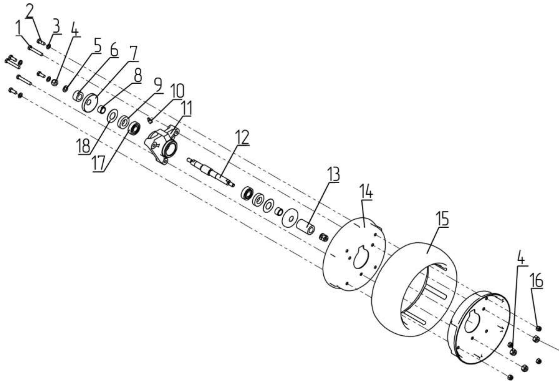
Рис.4 – Колесо КРН 46.090-Т
